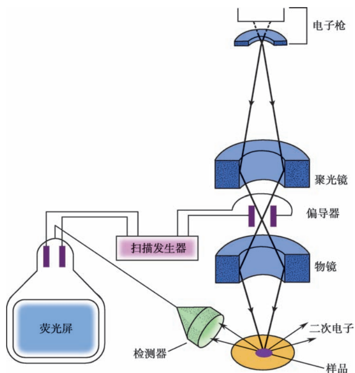
图 3-5 扫描电镜的工作原理
