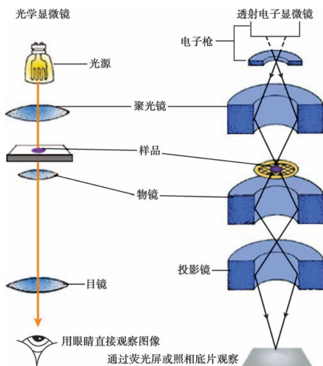
图 3-4 光学显微镜和透射电子显微镜的比较
