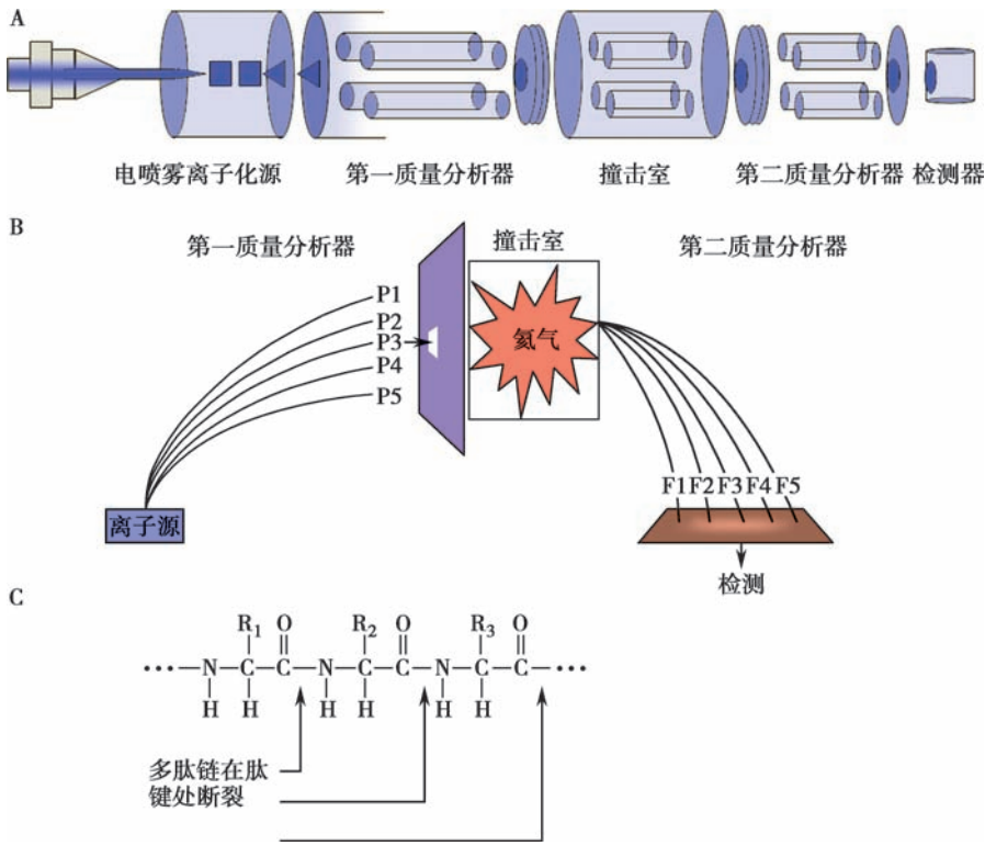
图 3-17 串联质谱测定多肽氨基酸序列
