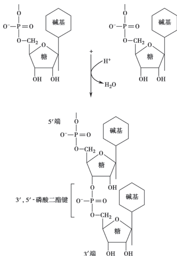
图 2-6 多核苷酸间的磷酸二酯键
