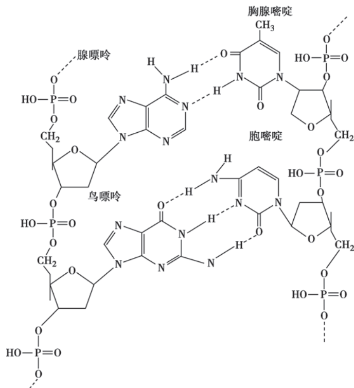
图 2-8 DNA 分子化学结构的一部分
