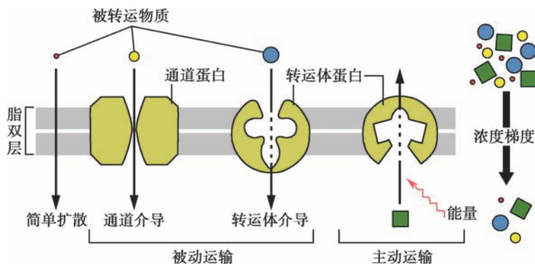
图 4-14 被动运输与主动运输
