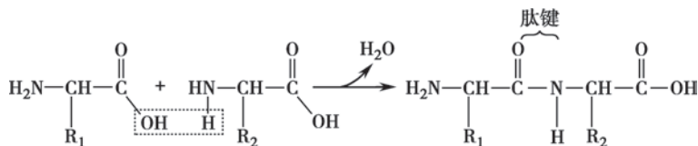
图 2-13 肽键的形成与结构
