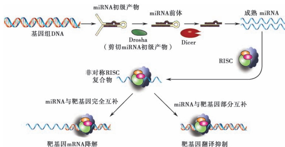
图 2-11 miRNA 的形成与作用机制
