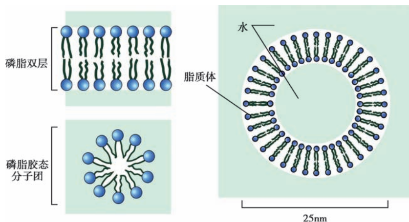
图 4-5 磷脂分子团和脂质体结构示意图
