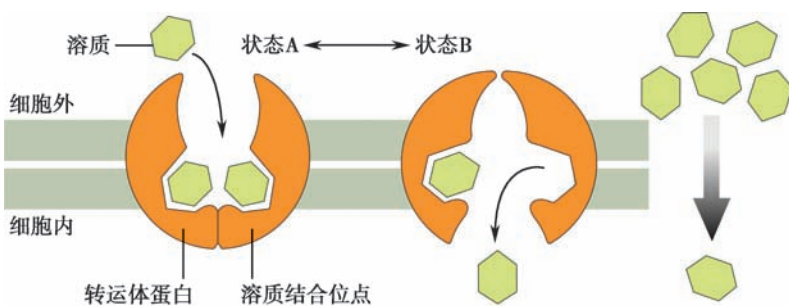
图 4-15 转运体蛋白构象变化介导的易化扩散示意图
