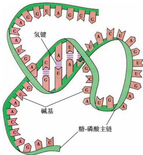
图 2-9 RNA 发夹结构模式图
