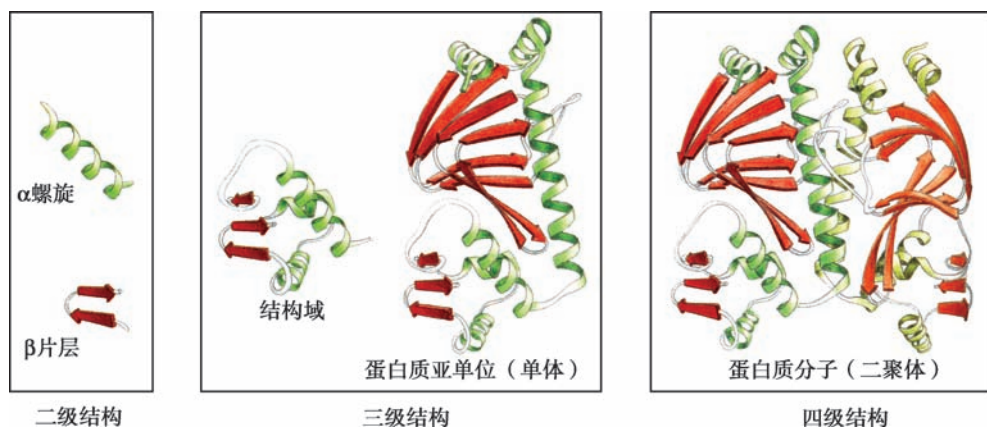
图 2-14 蛋白质分子高级结构示意图
