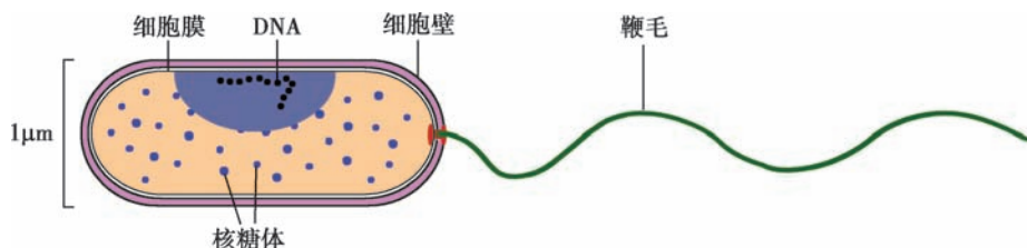
图 2-1 细菌结构示意图
