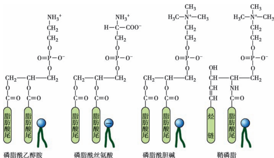
图 4-2 质膜中主要磷脂分子结构
