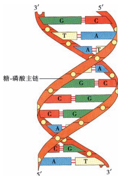
图 2-7 DNA 双螺旋结构模式图
