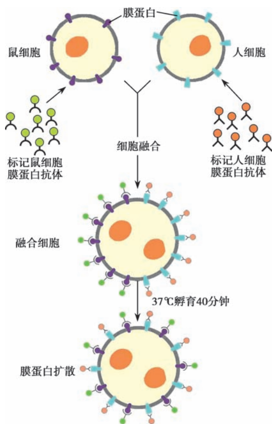
图 4-9 小鼠-人融合细胞膜蛋白侧向扩散示意图
