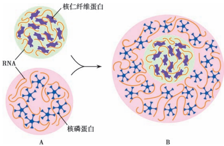
图 2-19 生物分子凝聚体的形成示意图
