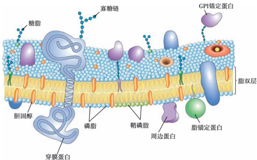
图 4-11 流动镶嵌模型
