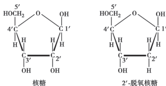
图 2-3 DNA 和 RNA 分子中戊糖的结构式
