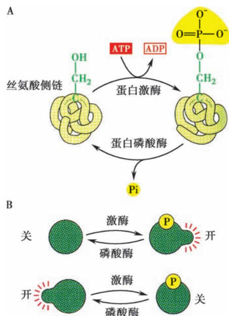
图 2-17 蛋白质的磷酸化与去磷酸调控其功能发挥
