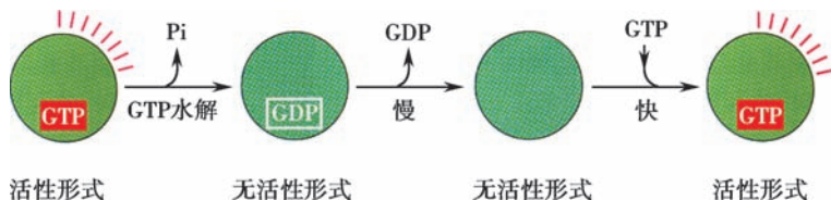
图 2-18 GTP 结合蛋白形成分子开关
