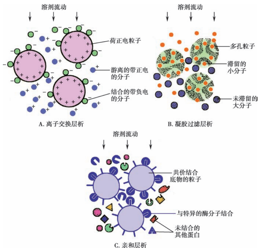
图 3-11 三种常用层析法的工作原理
