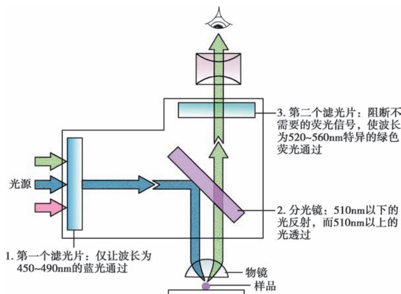
图 3-2 荧光显微镜的光学系统
