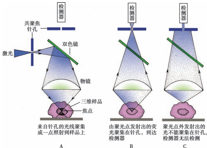
图 3-3 激光扫描共聚焦显微镜
