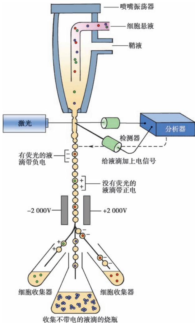
图 3-6 流式细胞仪原理图解
