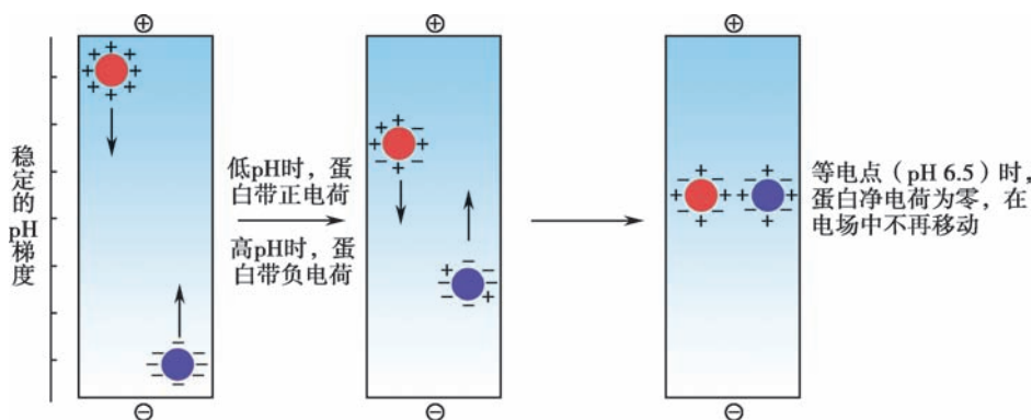
图 3-13 等电聚焦电泳分离蛋白质
