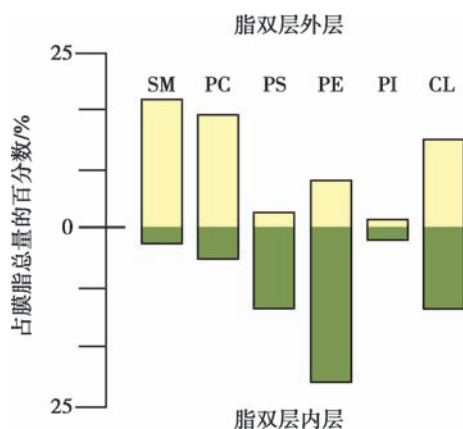
图 4-7 人红细胞膜中几种膜脂的不对称分布
