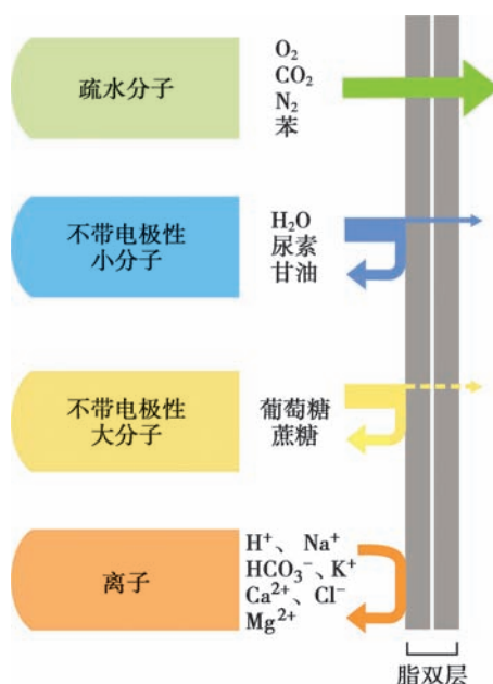
图 4-13 人工脂双层对不同溶质的相对通透性
