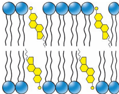
图 4-3 胆固醇与磷脂分子关系示意图 胆固醇亲水头部朝向脂双层的内外表面,大部分结构嵌入膜脂烃尾中并倾向于均匀分布。
