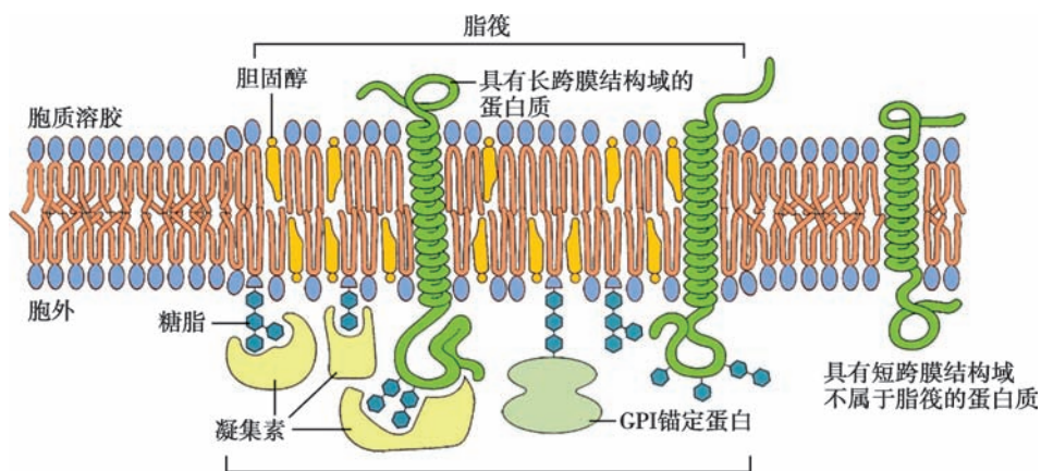
图 4-12 脂筏结构模式图
