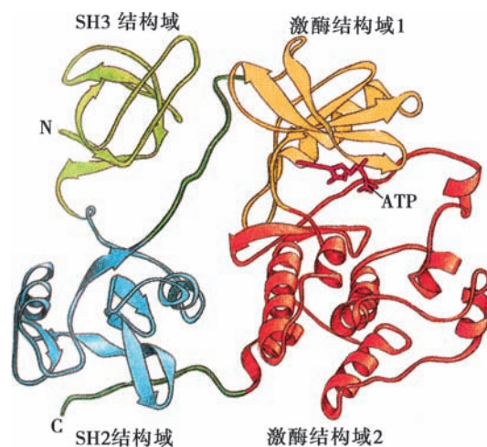
图 2-16 Src 蛋白的结构域
