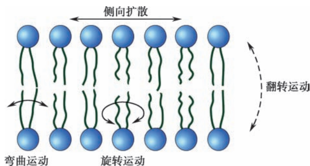
图4-8 膜脂分子的几种运动方式
