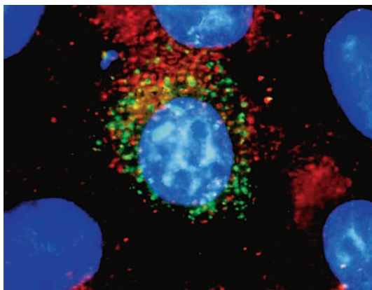
图3-14 辅酶Ⅱ依赖性视黄醇脱氢-还原酶选择性剪接体亚型(NRDRB1)在HeLa细胞中的定位 图中绿色荧光显示了N末端与GFP融合的NRDRB1在HeLa细胞内的分布,红色荧光是特异性标记的过氧化物酶体,两种颜色的荧光重叠处发出黄色荧光。该图说明NRDRB1仅有部分与过氧化物酶体重叠,从而定位到过氧化物酶体。
