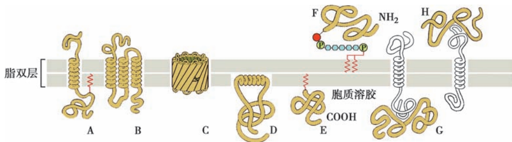
图 4-6 膜蛋白在膜中的几种结合方式
