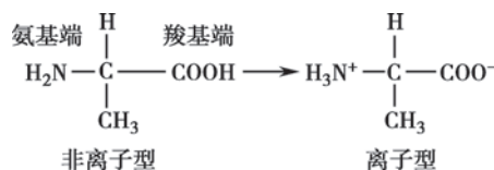
图 2-12 氨基酸的结构式
