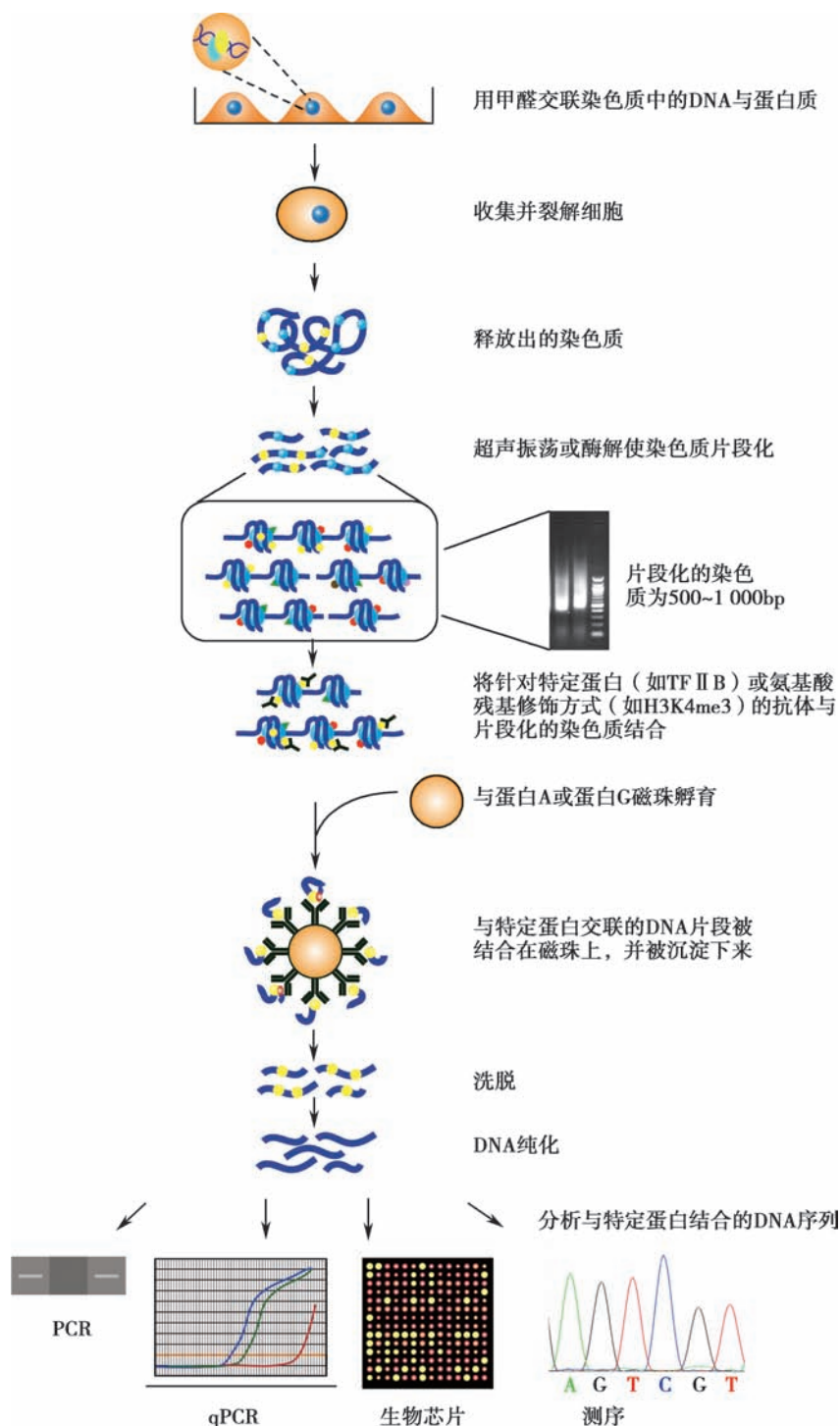
图 3-16 染色质免疫沉淀
