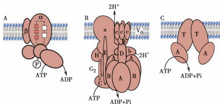
图 4-16 3 种类型 ATP 驱动泵模式图
