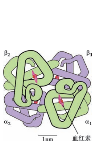
图 2-15 血红蛋白的四级结构
