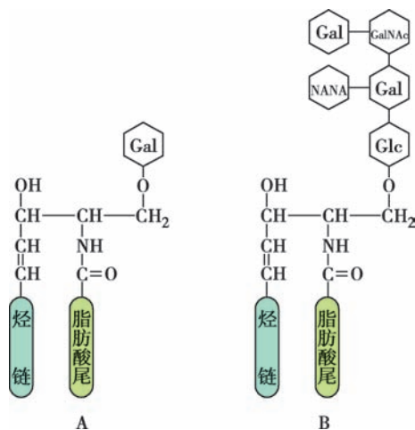
图 4-4 糖脂的化学结构
