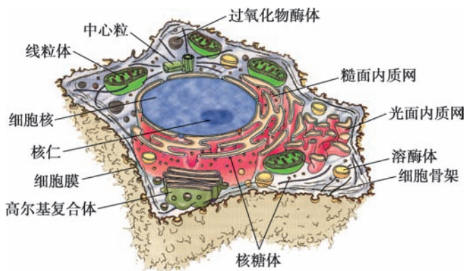
图 2-2 动物细胞结构模式图
