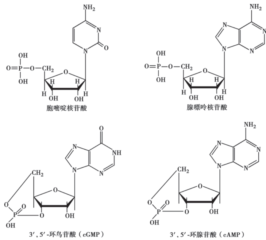
图 2-5 单核苷酸的结构式
