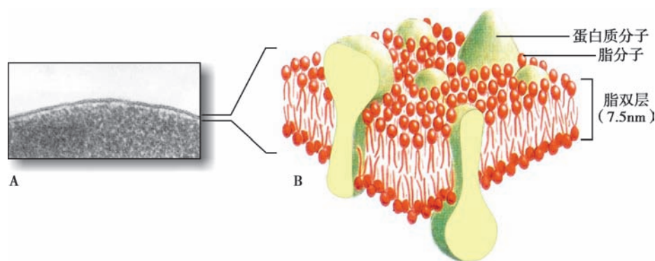
图 4-10 单位膜
