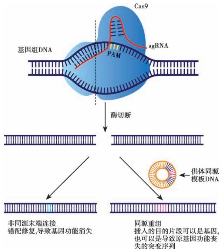
图 3-15 CRISPR/Cas9 技术
