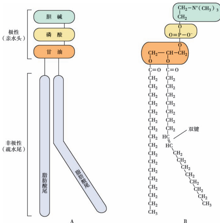
图 4-1 磷脂酰胆碱分子的结构
