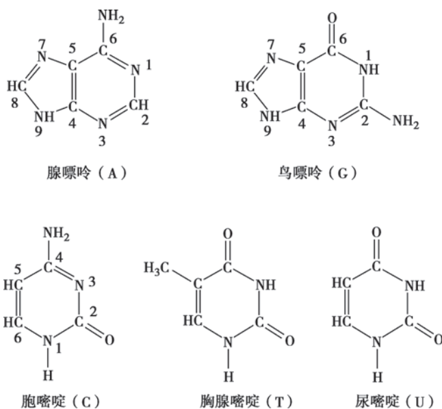
图 2-4 常见嘌呤和嘧啶的结构式
