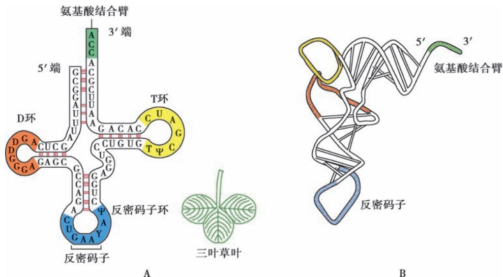
图 2-10 tRNA 的三叶草形结构
